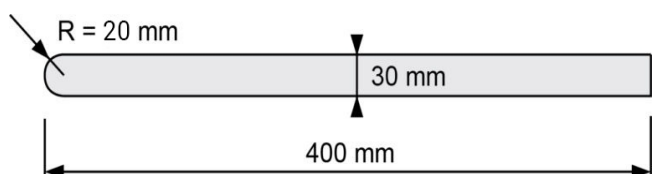
Schéma schodovky Granex® XXL 400 x 800 x 30 mm
